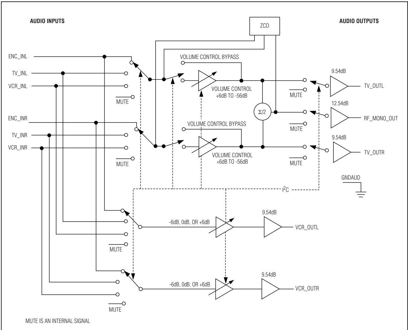
图4. MAX4397S 音频部分，具有单端编码器输入
