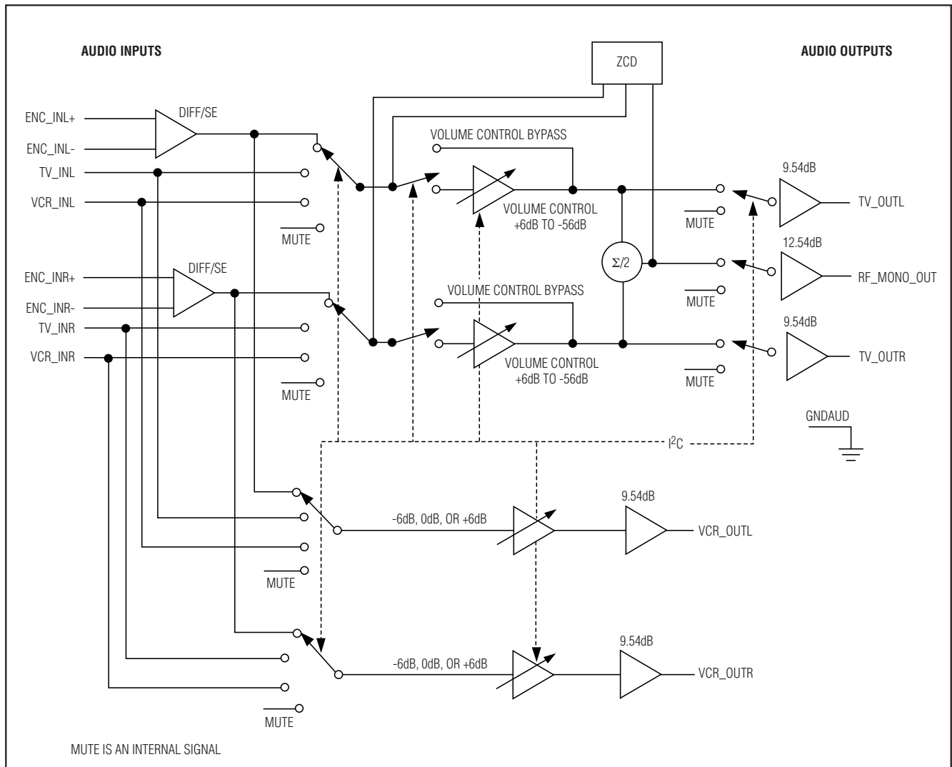
图3. MAX4397D 音频部分功能框图
