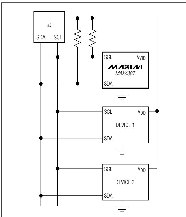
图6. 典型I 2 C接口应用
