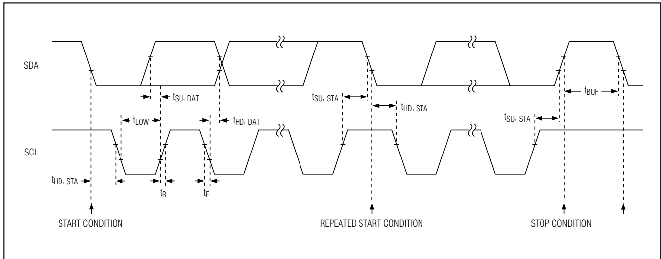
图5. SDA和SCL信号时序图
